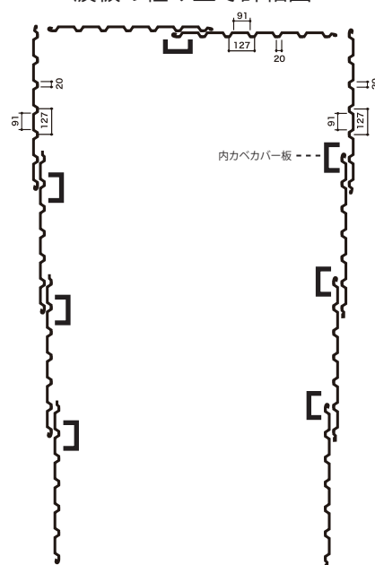
波板の組み立て詳細図
