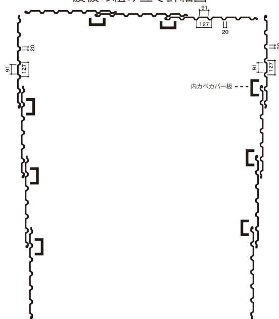
波板の組み立て詳細図
