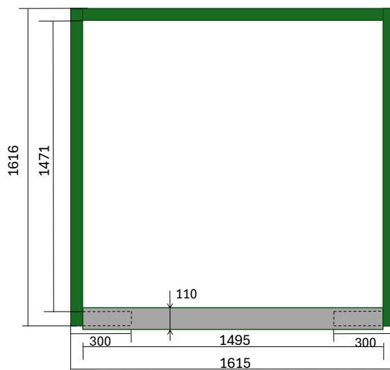
土台
