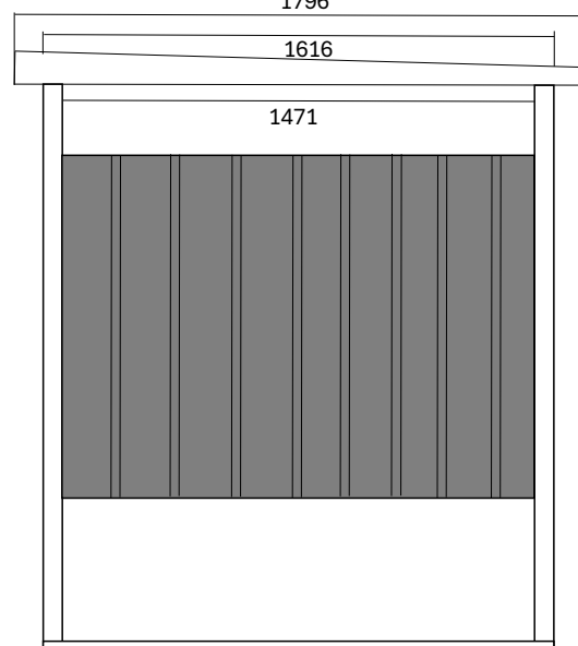
側面 1796
