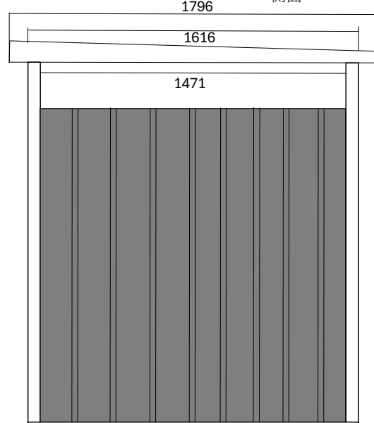
側面 1796
