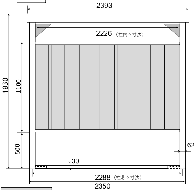
DM-10L・10LB
