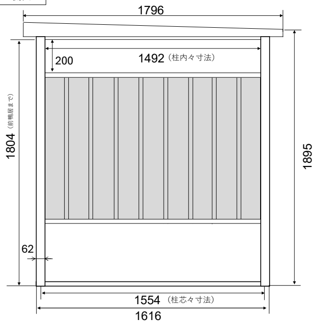
側面
