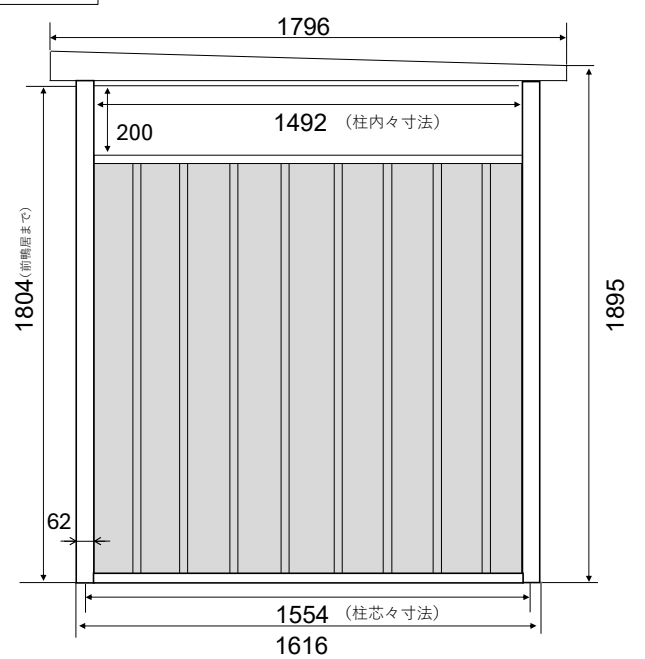
側面
