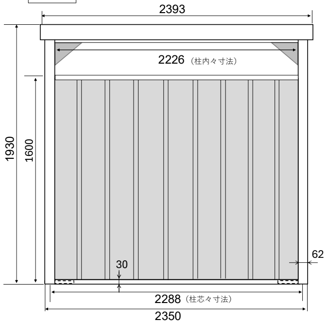
正面
