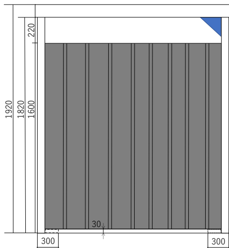
正面
