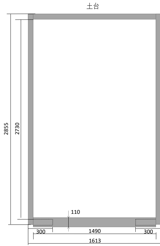
側面
